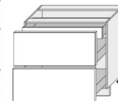
D2A/90/1A (900/820/500)
