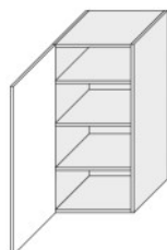
W4 40 (400/960/325)
