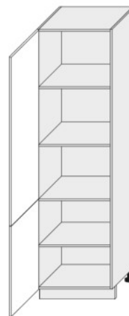
D14 DP 60 (600/2070/565)
