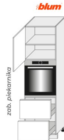
D14 RU 2M 60 356 L ● (600/2070/565)
