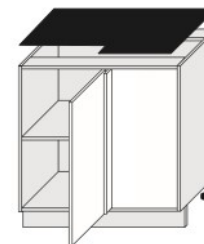
D13U 90 L/P (900/820/500)
