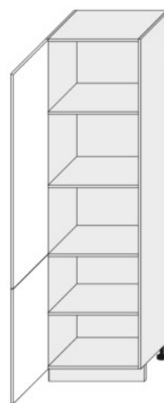
D14 DP 60 L/P (600/2070/565)
