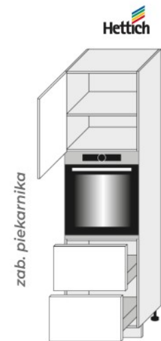
D14 RU 2A 60 356 L (600/2070/565)
