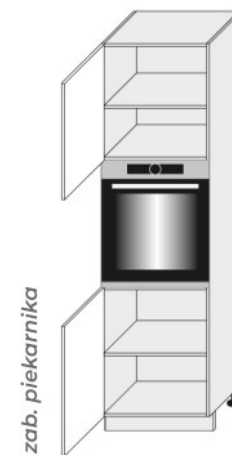
D14 RU 2D 60 L (600/2070/565)
