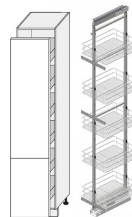
2D14K 40 + kosz MAXI 40 (400/2070/565)
