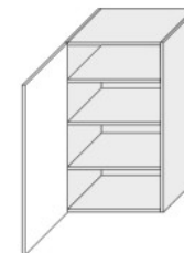
W4 60 (600/960/325)
