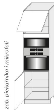
D14 RU 60 (600/2070/565)
