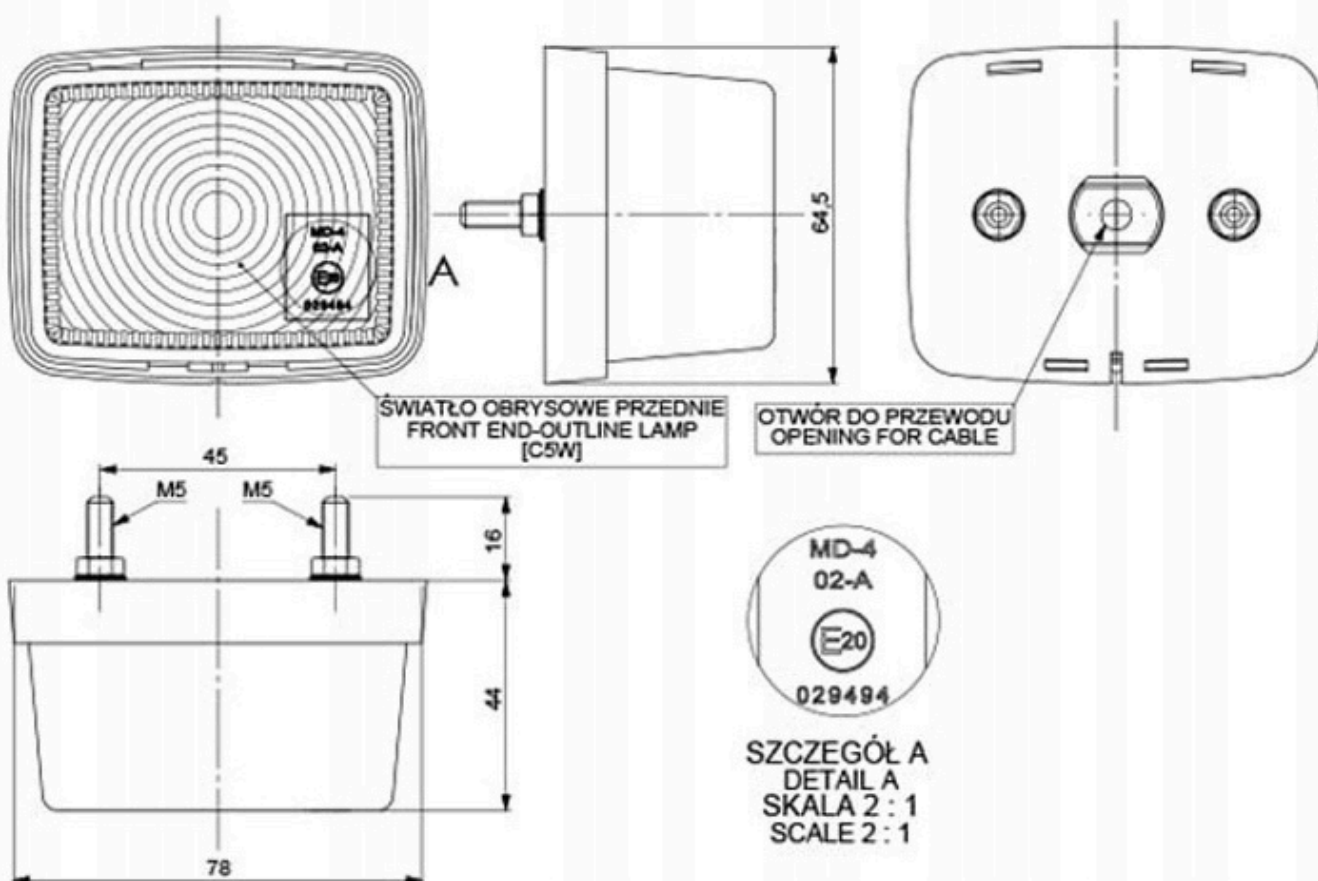
Lampa obrysowa prostokątna, biała [LO 208 ] Front rectangular end-outline lamp [ LO 208 ]
