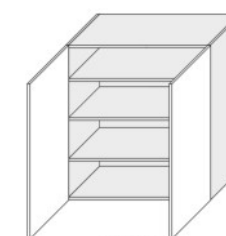
W4 90 (900/960/325)
