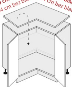
D12 90 P bez półki (840/820/840)
