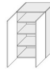
W4 60 2F (600/960/325)
