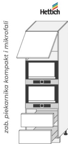
D14 RU 2A KOMPAKT (600/2070/565)
