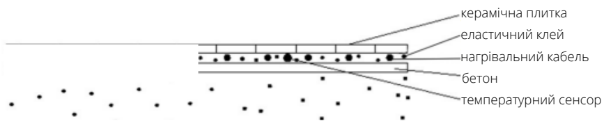
Малюнок 2: Безпосередньо на бетоні
