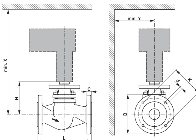
Rysunki wymiarowe
