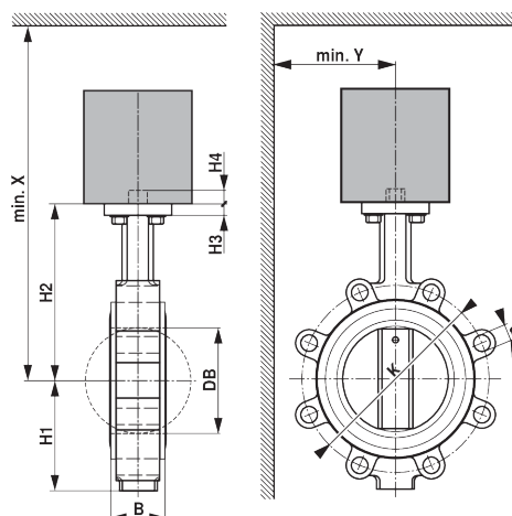
Rysunki wymiarowe
