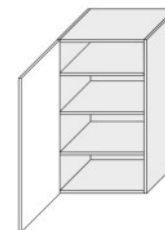
W4 50 L/P (500/960/325)
