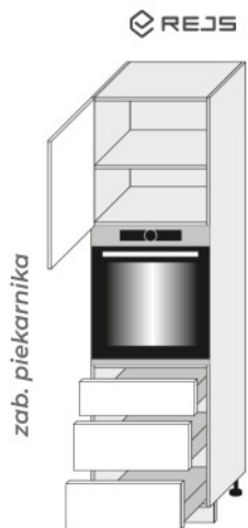
D14 RU 3R 60 L (600/2070/565)
