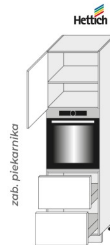
D14 RU 2A 60 356 L (600/2070/565)
