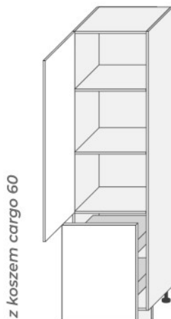
D14DP 60 L/P (600/2070/565)
