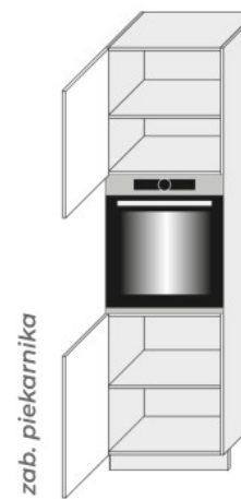
D14 RU 2D 60 (600/2070/565)
