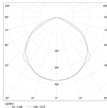
KANLUX S.A. (kat 25586) ANTRA LED100W-NW / Krzywa rozsyłu światła (biegunowo)
