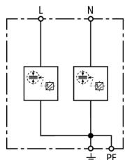
Schemat połączeń DSH TN 255
